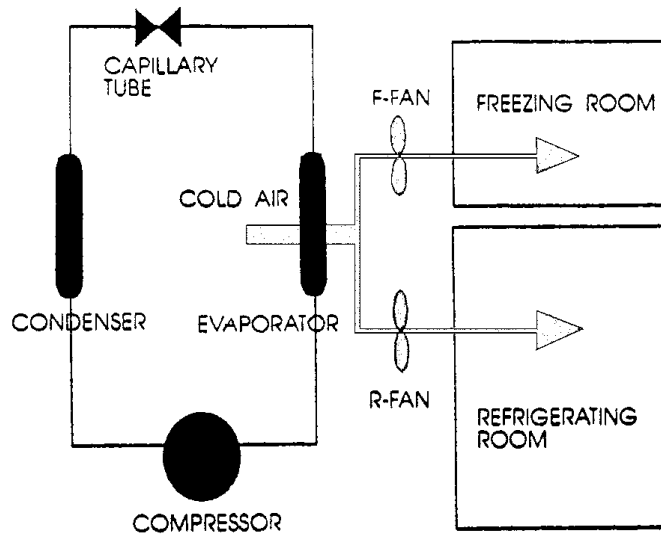
TWO COOLING FAN TYPE
